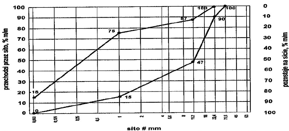
Rys. 4. Krzywe graniczne uziarnienia mieszanki kruszyw 0/22,4 mm do górnej warstwy podłoża ulepszzonego
